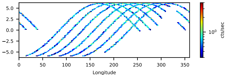
--saacalc=1 -saamode=STRICT --tentacle=yes 25.41-ks, 96%
