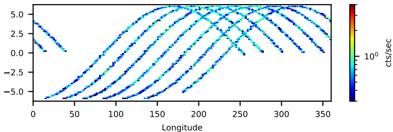
--saacalc=1 -saamode=STRICT --tentacle=no 25.41-ks, 96%
