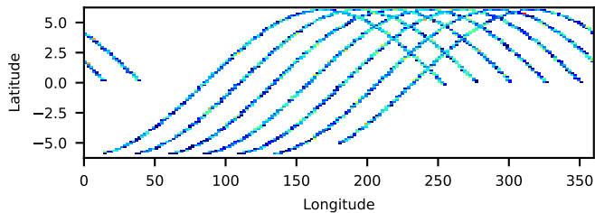
--saacalc=1 -saamode=OPTIMIZED --tentacle=no 26.54-ks, 100%
