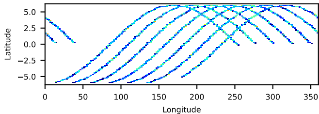
--saacalc=1 -saamode=OPTIMIZED --tentacle=yes 26.54-ks, 100%
