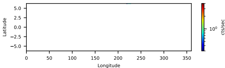
--saacalc=1 -saamode=OPTIMIZED --tentacle=no 0.13-ks, 100%
