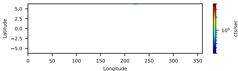
--saacalc=1 -saamode=OPTIMIZED --tentacle=yes 0.13-ks, 100%
