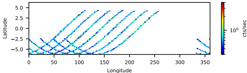
--saacalc=1 -saamode=OPTIMIZED --tentacle=yes 19.83-ks, 97%
