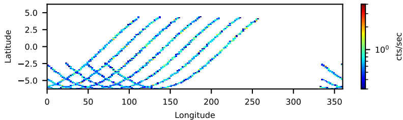
--saacalc=1 -saamode=OPTIMIZED --tentacle=no 19.83-ks, 97%
