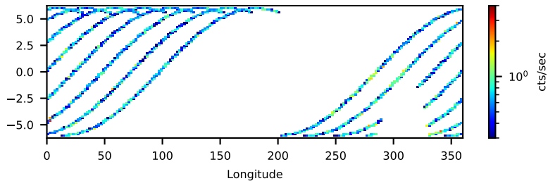
--saacalc=2 -saamode=OPTIMIZED --tentacle=no 21.55-ks, 98%
