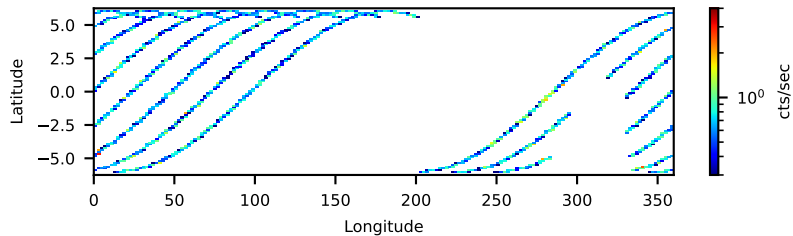
--saacalc=1 -saamode=OPTIMIZED --tentacle=no 21.23-ks, 97%
