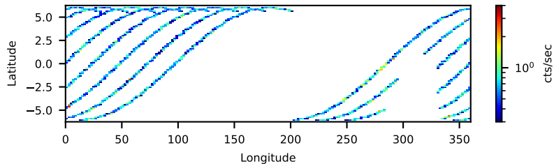
--saacalc=1 -saamode=OPTIMIZED --tentacle=yes 21.23-ks, 97%
