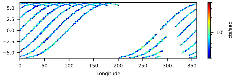
--saacalc=2 -saamode=OPTIMIZED --tentacle=yes 21.38-ks, 97%
