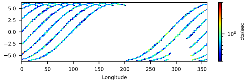
--saacalc=2 -saamode=STRICT --tentacle=no 16.19-ks, 74%
