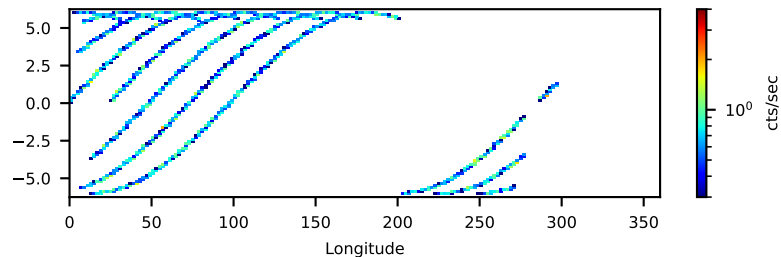
--saacalc=2 -saamode=STRICT --tentacle=yes 16.03-ks, 73%
