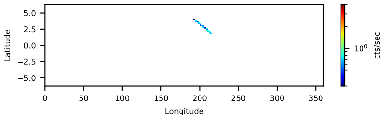
--saacalc=1 -saamode=OPTIMIZED --tentacle=yes 0.34-ks, 100%
