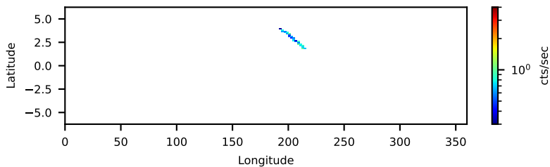
--saacalc=1 -saamode=OPTIMIZED --tentacle=no 0.34-ks, 100%
