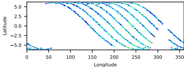
--saacalc=1 -saamode=OPTIMIZED --tentacle=yes 22.24-ks, 98%
