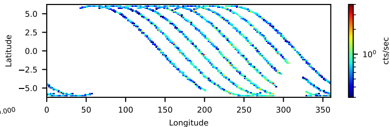
--saacalc=3 -saamode=STRICT --tentacle=no 19.19-ks, 84%
