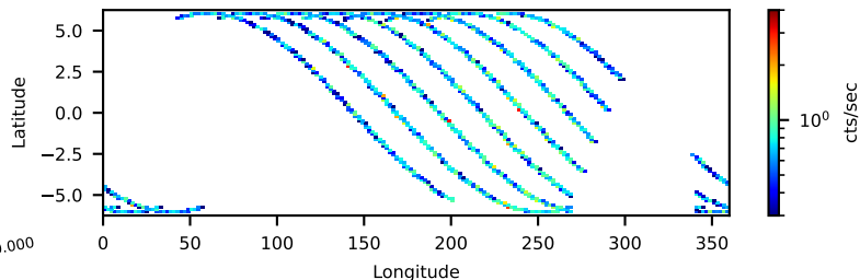
--saacalc=1 -saamode=STRICT --tentacle=yes 20.42-ks, 90%
