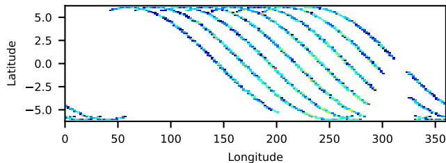
--saacalc=1 -saamode=OPTIMIZED --tentacle=no 22.24-ks, 98%
