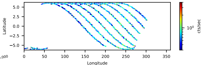
--saacalc=3 -saamode=STRICT --tentacle=yes 19.19-ks, 84%
