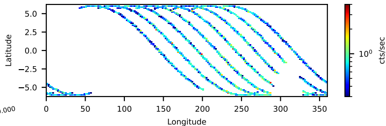
--saacalc=1 -saamode=STRICT --tentacle=no 20.42-ks, 90%
