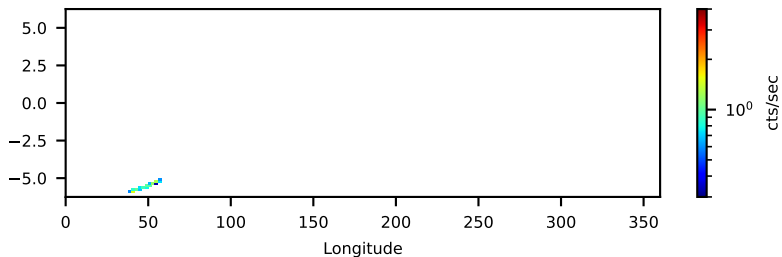
--saacalc=3 -saamode=OPTIMIZED --tentacle=no 0.29-ks, 100%
