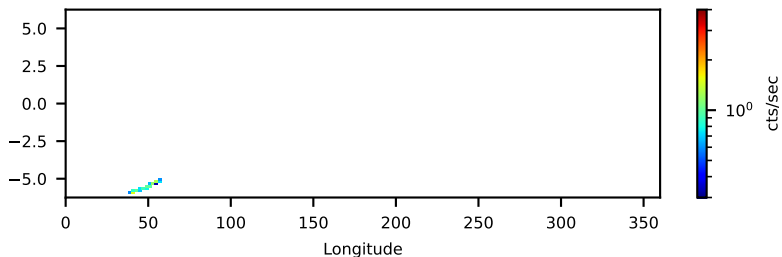
--saacalc=3 -saamode=OPTIMIZED --tentacle=yes 0.29-ks, 100%
