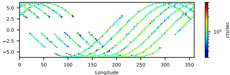
--saacalc=1 -saamode=STRICT --tentacle=no 25.19-ks, 90%
