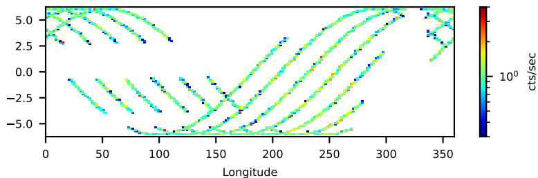
--saacalc=1 -saamode=STRICT --tentacle=yes 25.19-ks, 90%
