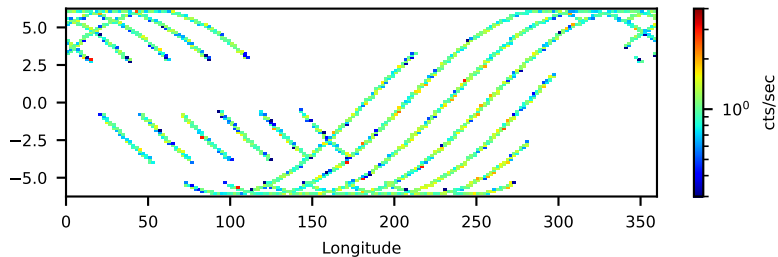
--saacalc=2 -saamode=STRICT --tentacle=yes 25.26-ks, 90%
