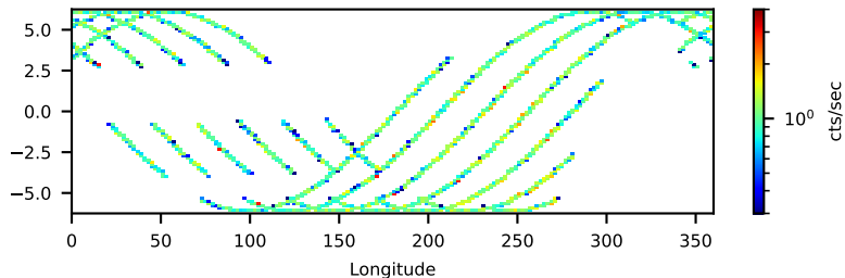
--saacalc=3 -saamode=STRICT --tentacle=yes 25.26-ks, 90%
