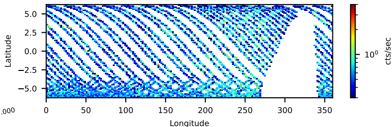
--saacalc=1 -saamode=STRICT --tentacle=yes 95.39-ks, 91%
