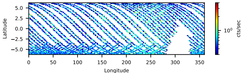
--saacalc=1 -saamode=OPTIMIZED --tentacle=yes 102.41-ks, 98%
