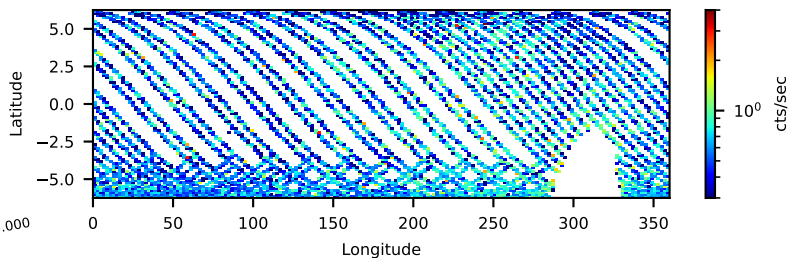
--saacalc=1 -saamode=STRICT --tentacle=no 95.39-ks, 91%
