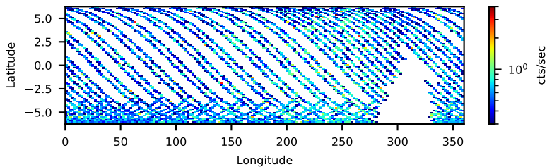
--saacalc=1 -saamode=OPTIMIZED --tentacle=no 102.41-ks, 98%
