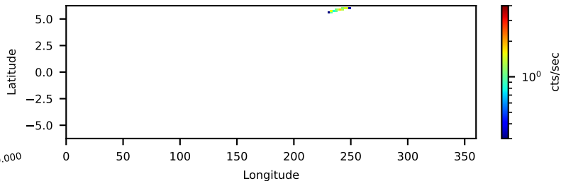
--saacalc=1 -saamode=STRICT --tentacle=no 0.27-ks, 100%
