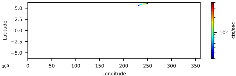
--saacalc=1 -saamode=STRICT --tentacle=yes 0.27-ks, 100%
