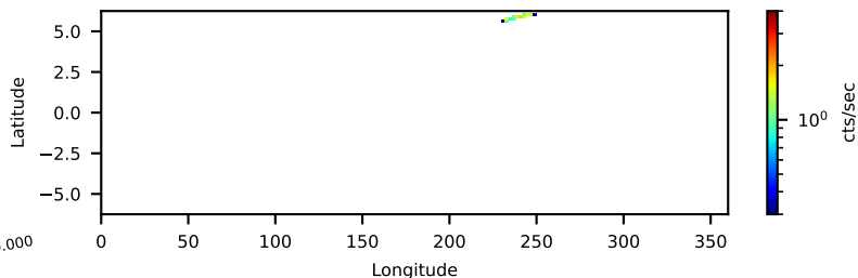
--saacalc=3 -saamode=OPTIMIZED --tentacle=yes 0.27-ks, 100%
