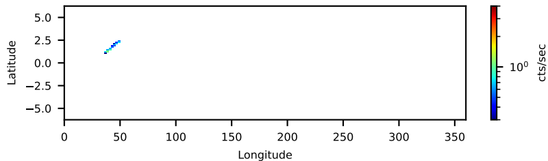
--saacalc=1 -saamode=OPTIMIZED --tentacle=yes 0.21-ks, 100%
