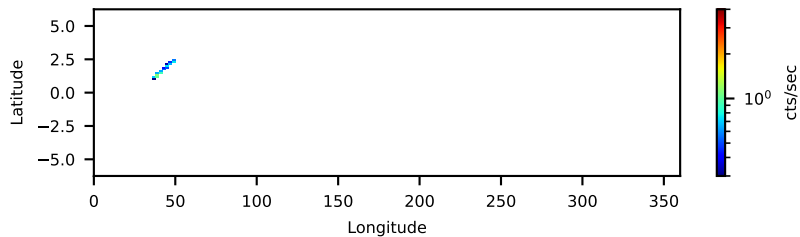
--saacalc=1 -saamode=OPTIMIZED --tentacle=no 0.21-ks, 100%
