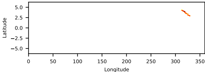
--saacalc=1 -saamode=OPTIMIZED --tentacle=yes 0.26-ks, 100%
