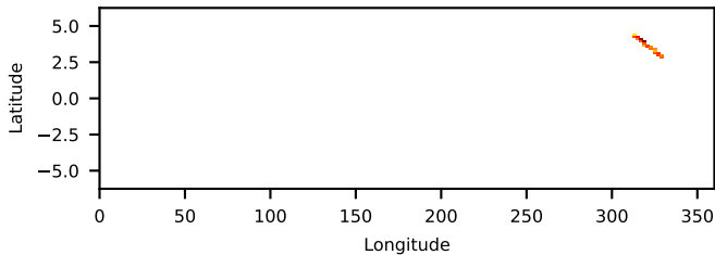
--saacalc=1 -saamode=OPTIMIZED --tentacle=no 0.26-ks, 100%
