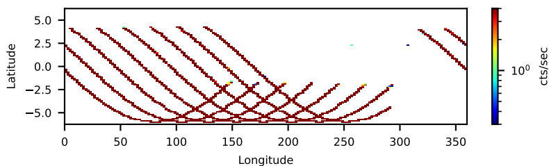
--saacalc=1 -saamode=OPTIMIZED --tentacle=no 22.88-ks, 100%
