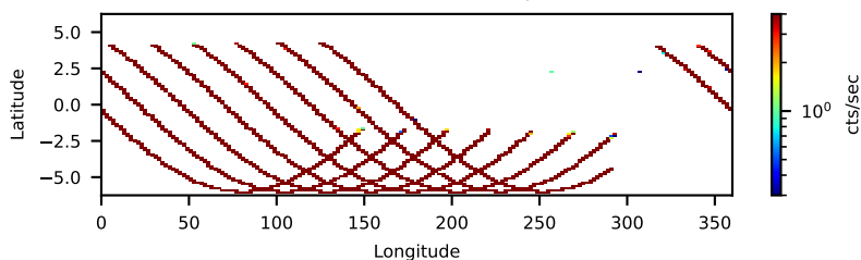
--saacalc=1 -saamode=OPTIMIZED --tentacle=yes 22.88-ks, 100%
