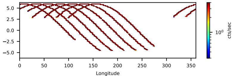
--saacalc=3 -saamode=STRICT --tentacle=yes 19.11-ks, 98%
