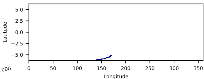
91002519001: 30 to 120 keV
