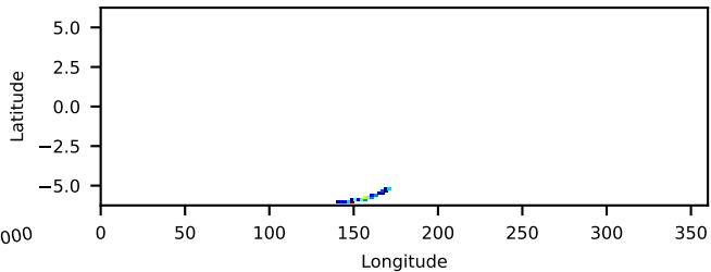
91002519001: 3 to 10 keV
