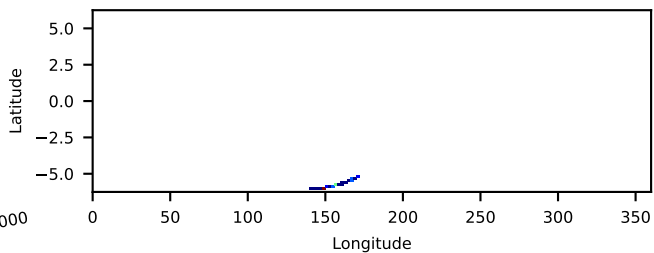
91002519001: 30 to 120 keV
