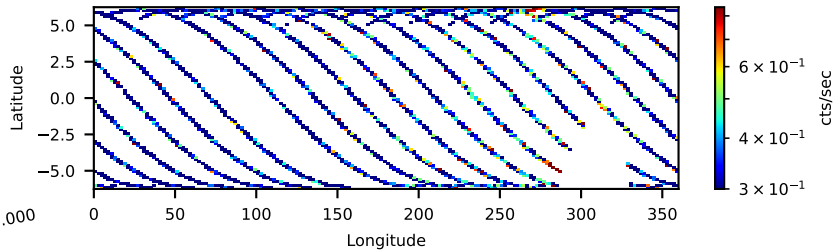
90902520002: 30 to 120 keV
