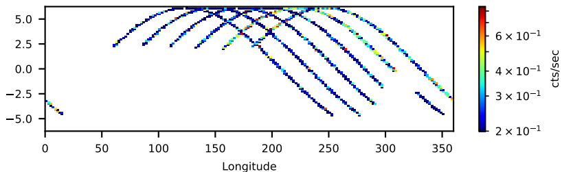
90902326006: 30 to 120 keV
