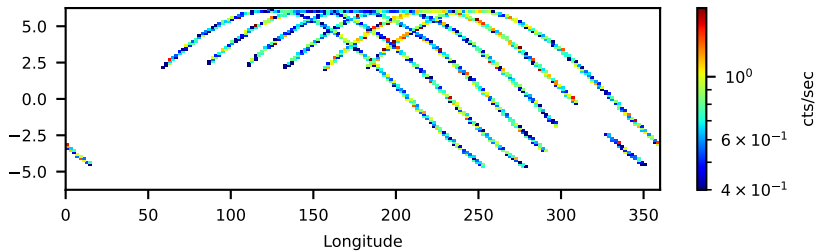
90902326006: 3 to 10 keV
