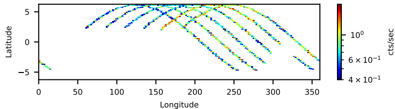
90902326006: 3 to 120 keV
