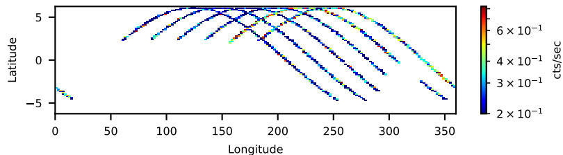
90902326006: 3 to 10 keV
