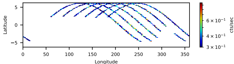
90902326006: 30 to 120 keV
