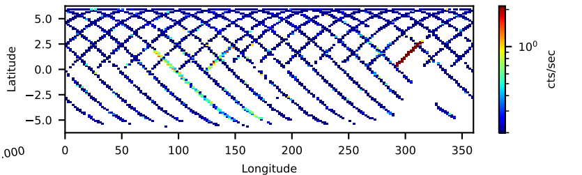
90902319002: 30 to 120 keV
