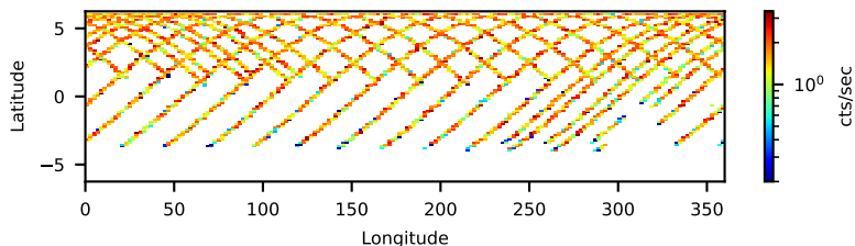
90901313002: 3 to 10 keV
