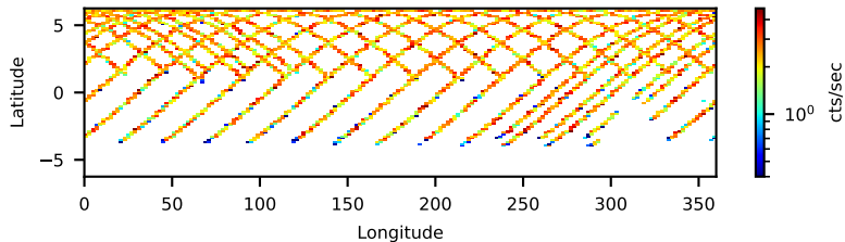
90901313002: 3 to 120 keV
