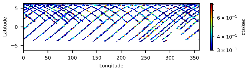
90901313002: 30 to 120 keV
