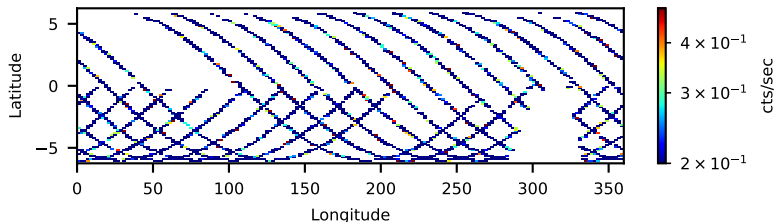
90901301004: 3 to 10 keV
