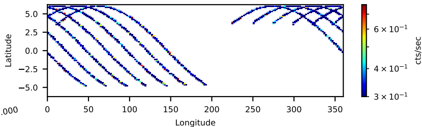
90802013006: 30 to 120 keV
