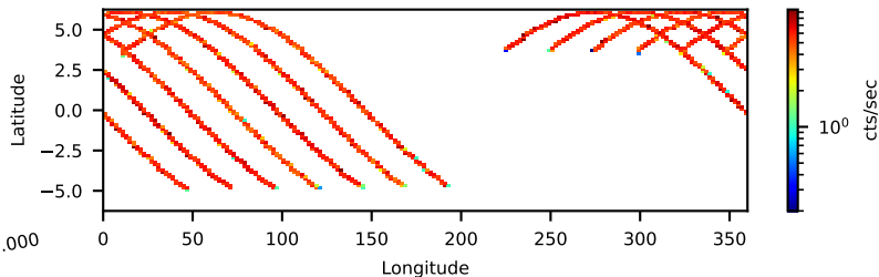
90802013006: 30 to 120 keV
