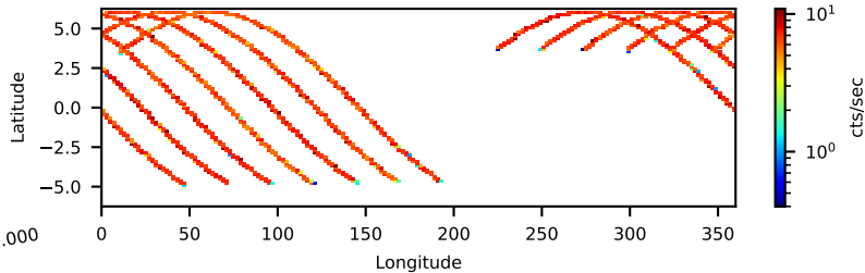
90802013006: 3 to 10 keV
