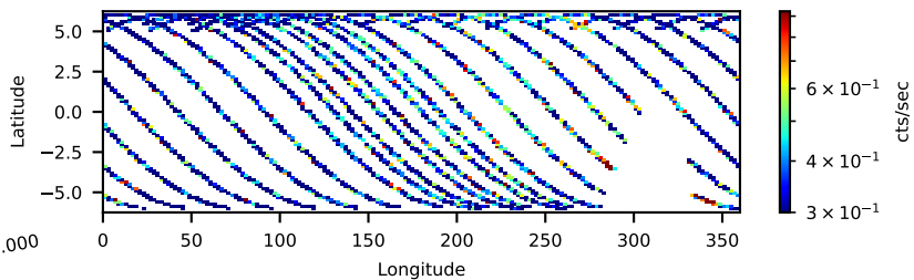
90801617002: 30 to 120 keV
