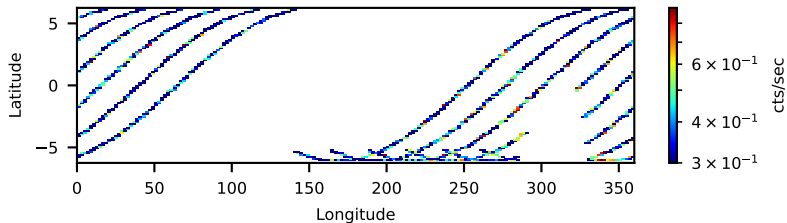
90801535006: 30 to 120 keV
