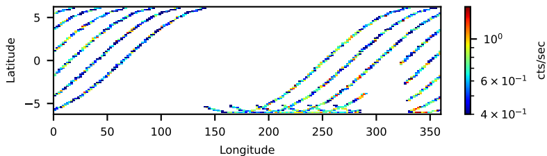
90801535006: 3 to 120 keV
