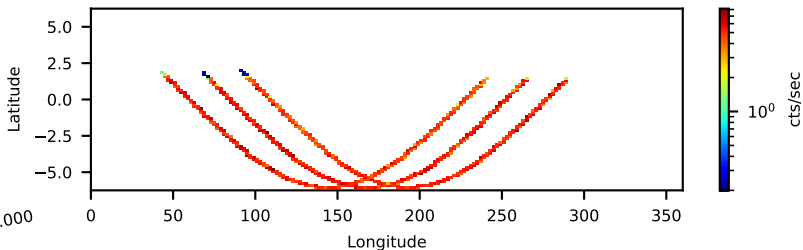
90801022002: 30 to 120 keV
