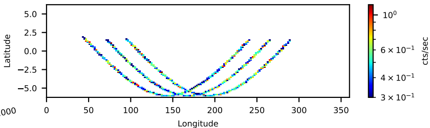
90801022002: 30 to 120 keV
