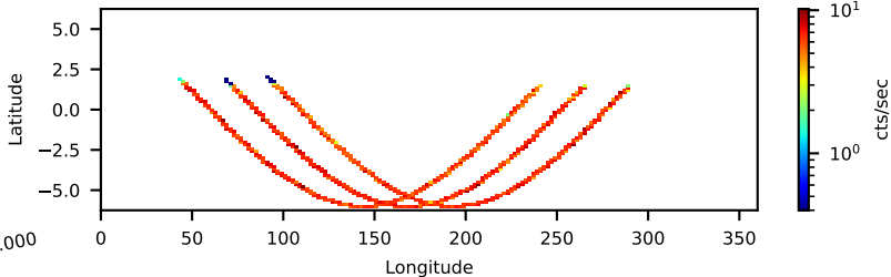
90801022002: 3 to 10 keV
