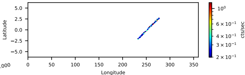
90801015002: 30 to 120 keV
