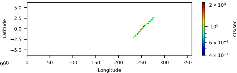
90801015002: 3 to 10 keV
