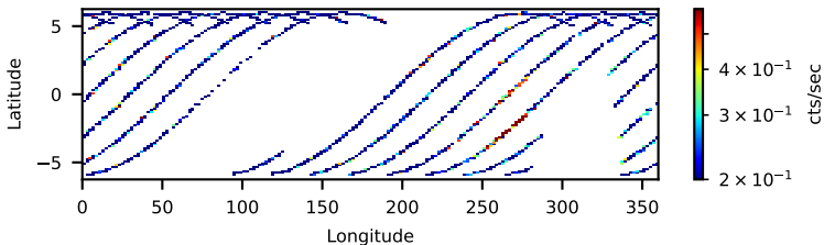
90602619006: 3 to 10 keV
