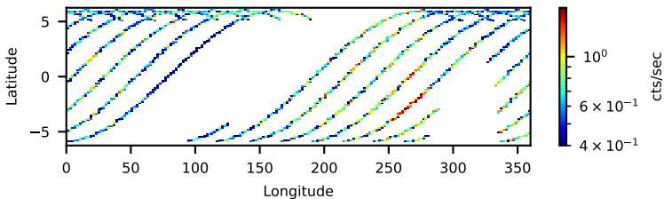
90602619006: 3 to 120 keV
