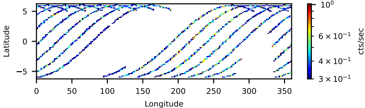
90602619006: 30 to 120 keV
