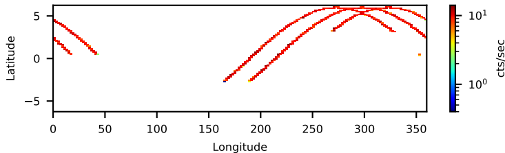
90302319006: 3 to 120 keV
