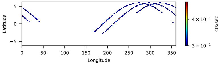
90302319006: 30 to 120 keV
