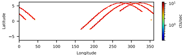
90302319006: 3 to 10 keV
