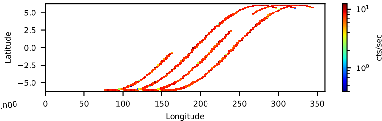
90302319004: 3 to 10 keV
