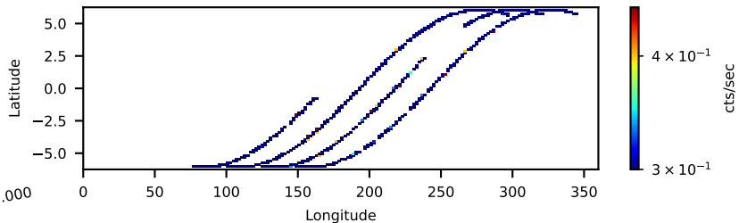
90302319004: 30 to 120 keV
