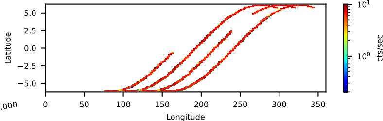
90302319004: 30 to 120 keV
