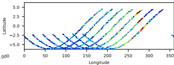
90301618004: 3 to 10 keV
