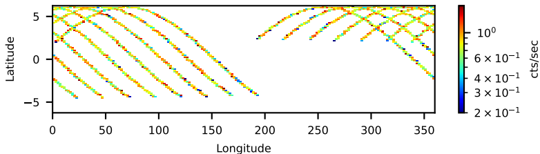
90202052002: 3 to 10 keV
