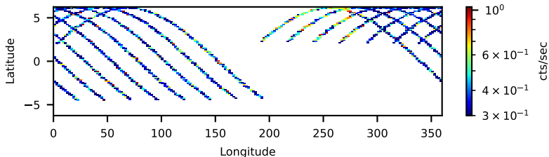
90202052002: 30 to 120 keV
