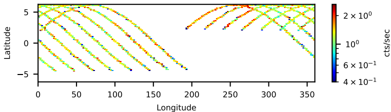
90202052002: 3 to 120 keV
