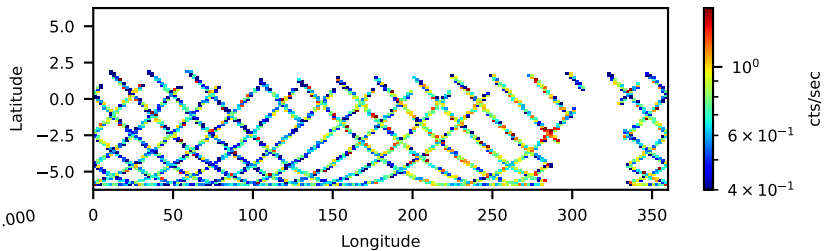
90201057002: 3 to 10 keV
