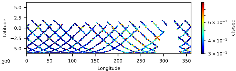
90201057002: 30 to 120 keV
