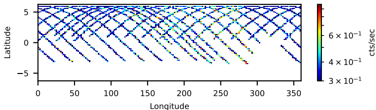
90201043002: 30 to 120 keV
