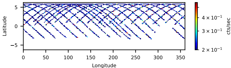
90201043002: 3 to 10 keV
