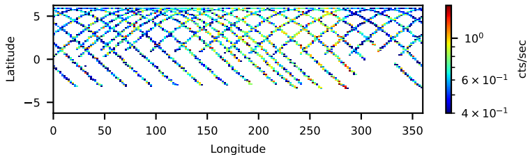
90201043002: 3 to 120 keV
