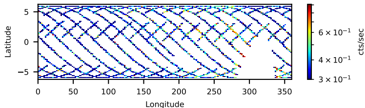
90201023002: 30 to 120 keV
