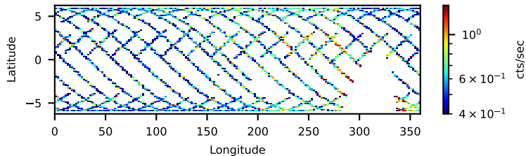
90201023002: 3 to 120 keV
