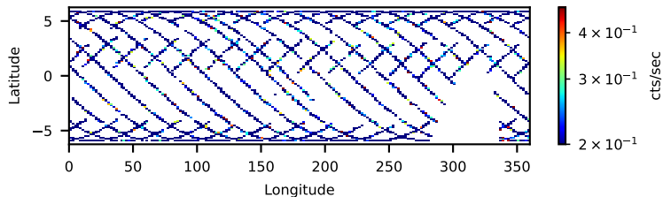
90201023002: 3 to 10 keV
