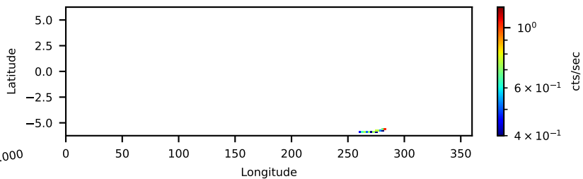
90201023001: 3 to 10 keV
