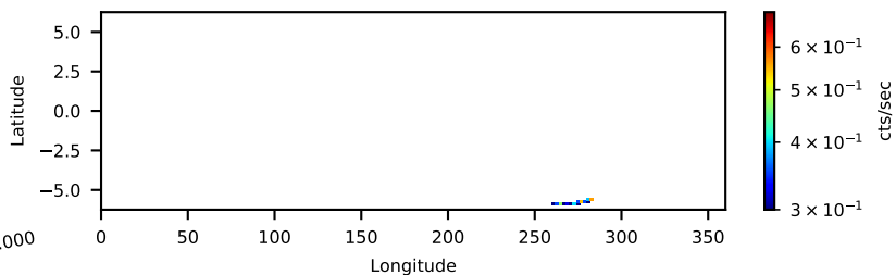
90201023001: 30 to 120 keV
