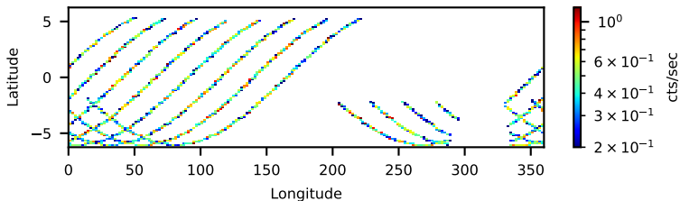
90001003002: 3 to 10 keV
