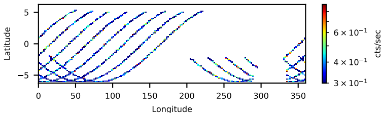
90001003002: 30 to 120 keV
