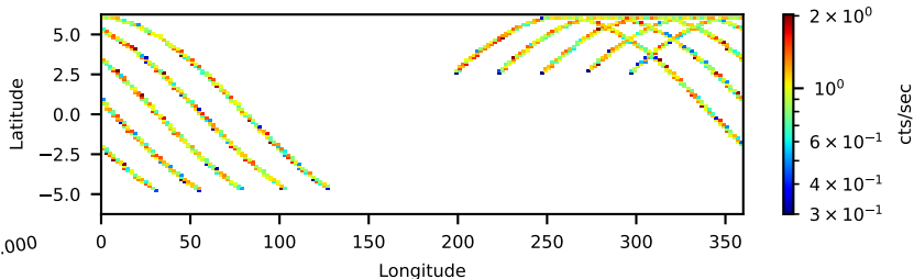
80902013006: 30 to 120 keV
