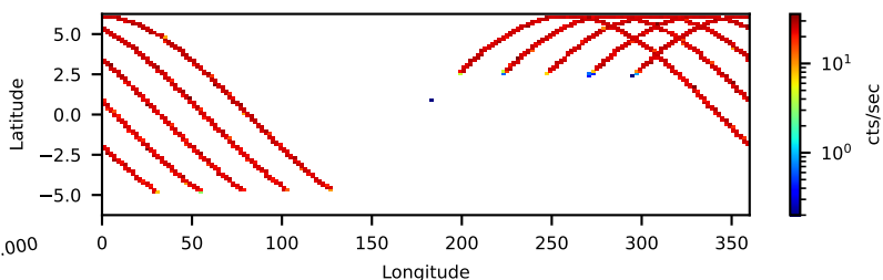
80902013006: 30 to 120 keV
