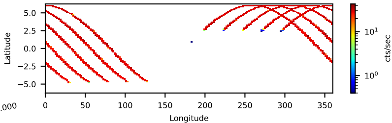
80902013006: 3 to 10 keV
