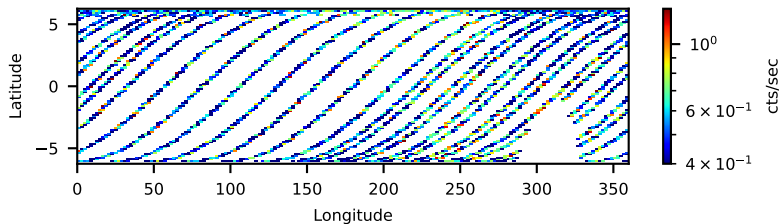
80802652004: 3 to 120 keV
