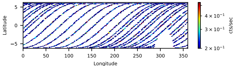
80802652004: 3 to 10 keV
