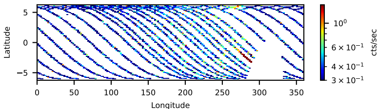
80801603002: 30 to 120 keV
