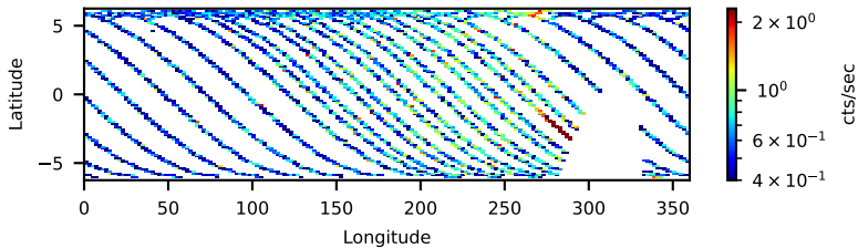
80801603002: 3 to 120 keV
