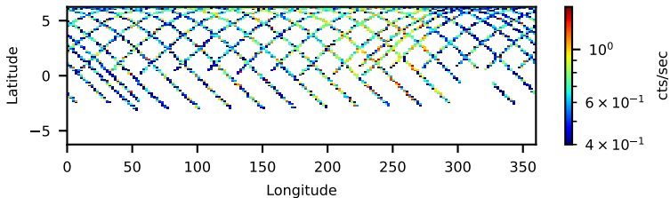
80702508004: 3 to 120 keV
