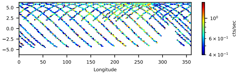
80702311002: 3 to 10 keV
