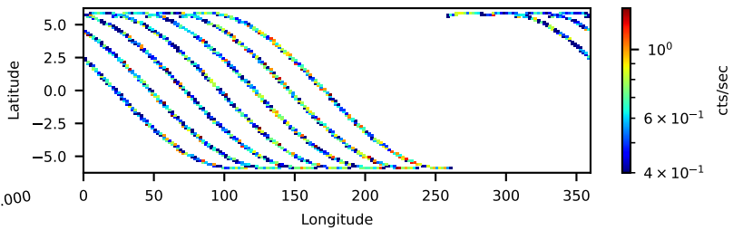
80701621002: 3 to 10 keV
