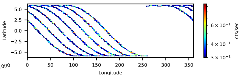
80701621002: 30 to 120 keV
