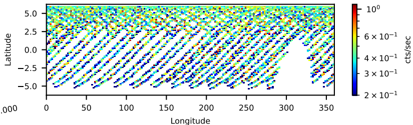
80701312002: 30 to 120 keV
