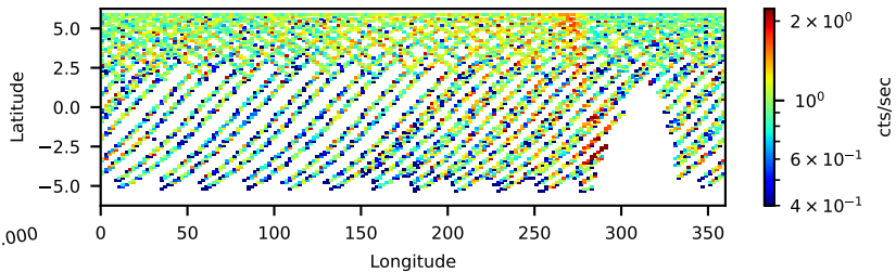
80701312002: 3 to 10 keV
