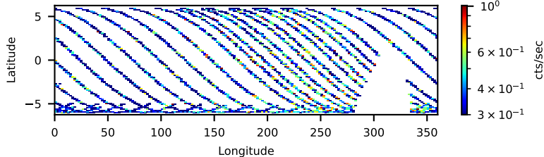
80602604002: 30 to 120 keV
