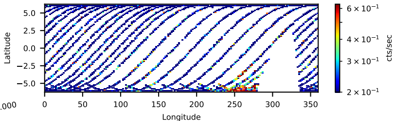
80601317002: 30 to 120 keV
