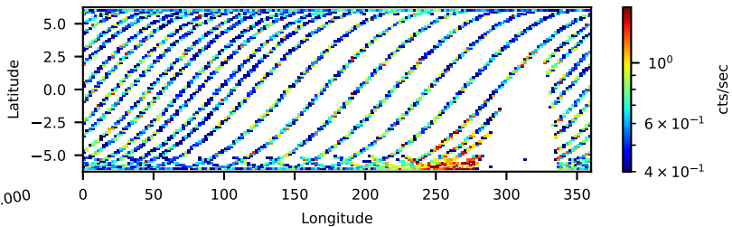
80601317002: 3 to 10 keV
