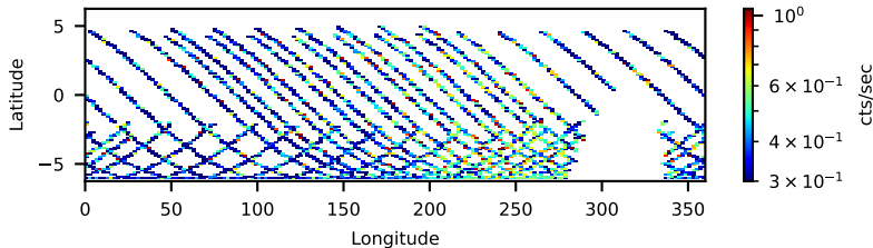
80502515002: 30 to 120 keV
