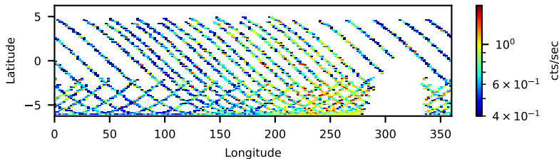
80502515002: 3 to 120 keV
