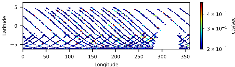
80502515002: 3 to 10 keV
