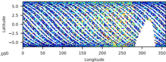
80502407002: 3 to 10 keV
