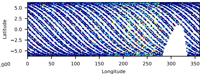
80502407002: 30 to 120 keV
