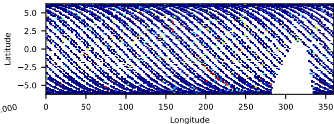
80502407002: 30 to 120 keV
