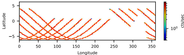
80502304004: 3 to 120 keV
