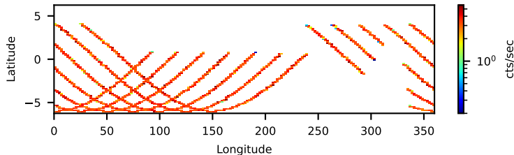
80502304004: 3 to 10 keV
