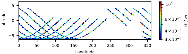
80502304004: 30 to 120 keV
