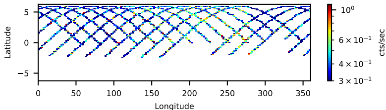
80401424002: 30 to 120 keV
