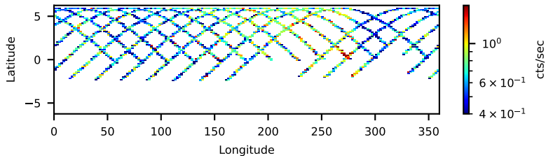
80401424002: 3 to 120 keV
