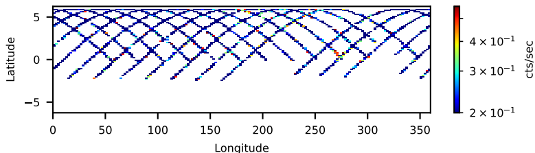
80401424002: 3 to 10 keV
