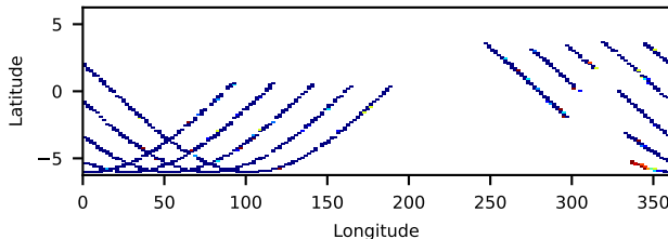
80302309006: 30 to 120 keV
