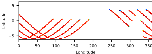
80302309006: 3 to 10 keV
