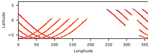
80302309006: 3 to 120 keV
